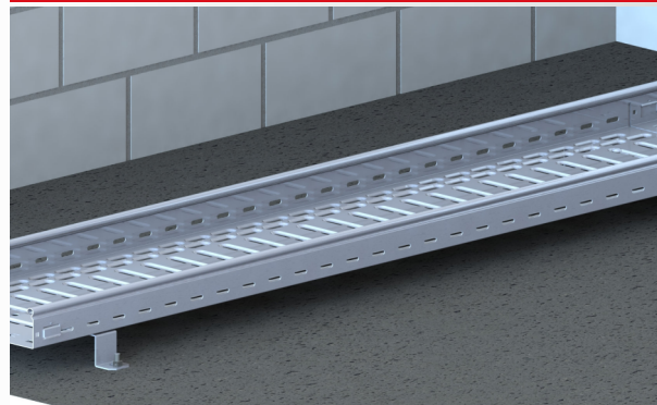
Montaža regala na odstoynik vrši se pomoću torban vijaka tipa PEKOM M6x12
