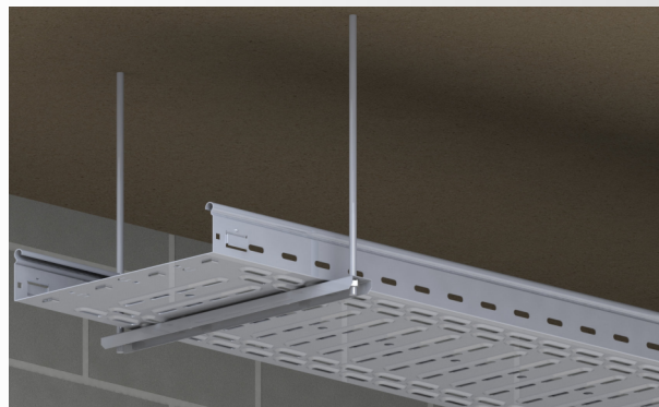
Za montažu regala na plafon pomoću dve navojne šipke, koristi se profilna perforirana šina
