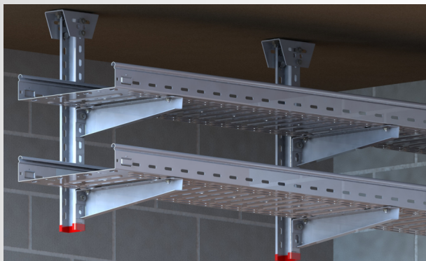
Plafonska montaža regala u više nivoa vrši se pomoću UD nosača, U profila i konzola
