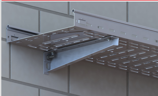
Pričvršćivanje nosača kablova za konzolu vrši se torban vijcima PEKOM M6x12
